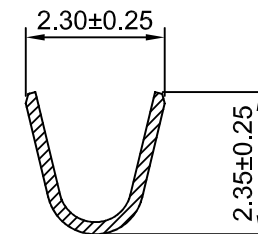
SEC:A-A
